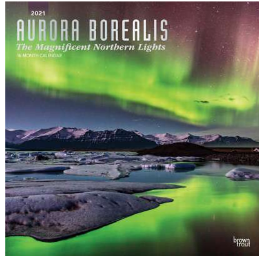
AURORA BOREALIS
